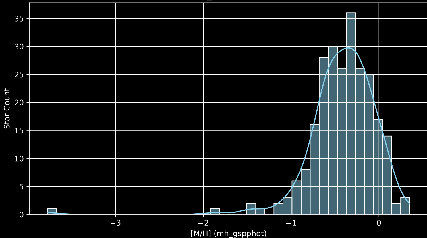
GALAH DR4 Field: [9217] [M/H] (mh_gspphot) (n= 247)
