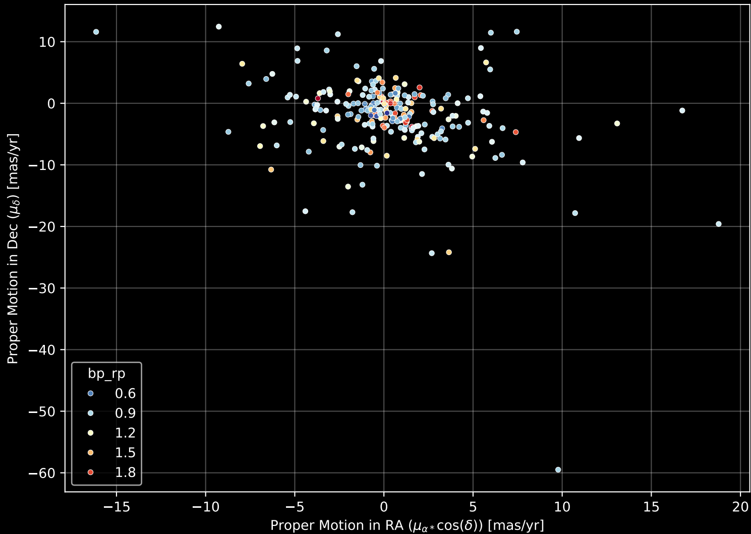
GALAH DR4 Field: [9217] Proper Motion Diagram (n= 247)
