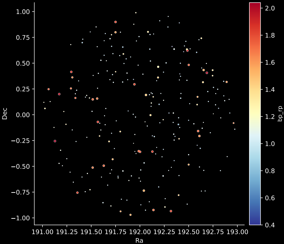
GALAH DR4 Field: [9217] Stars: 247
