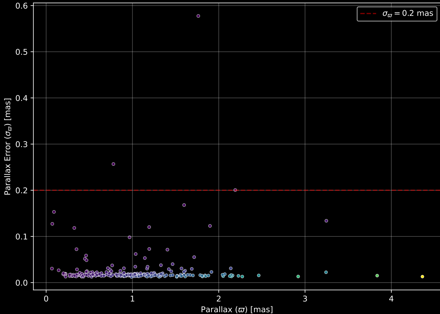
GALAH DR4 Field: [9217] Parallax Quality (n= 247)
