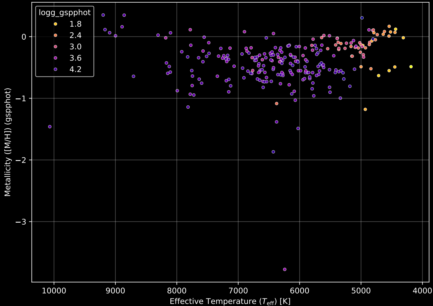
GALAH DR4 Field: [9217] Stellar Population Parameters (n= 247)
